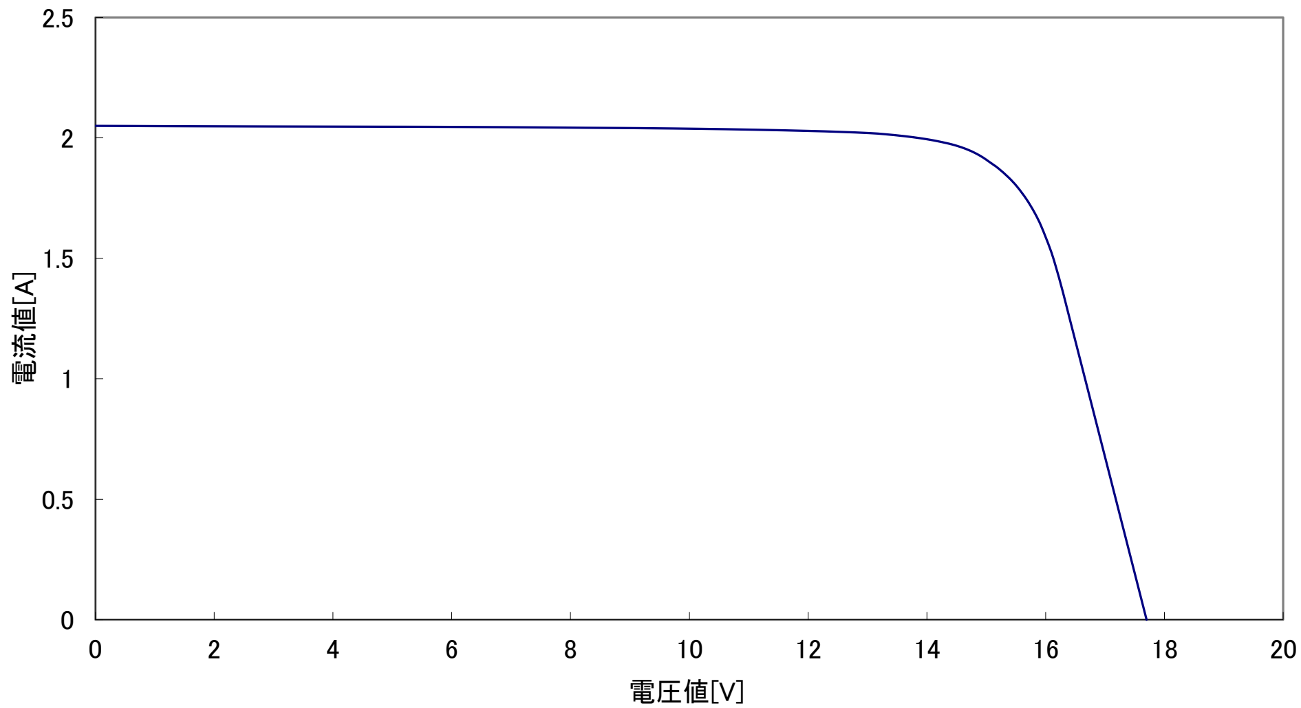
GT230S 出力特性図 @1000W/m 2 AM1.5 25°C
